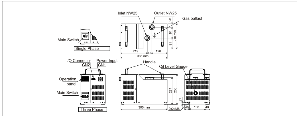
PumpSchematics(NeoDry15C)
