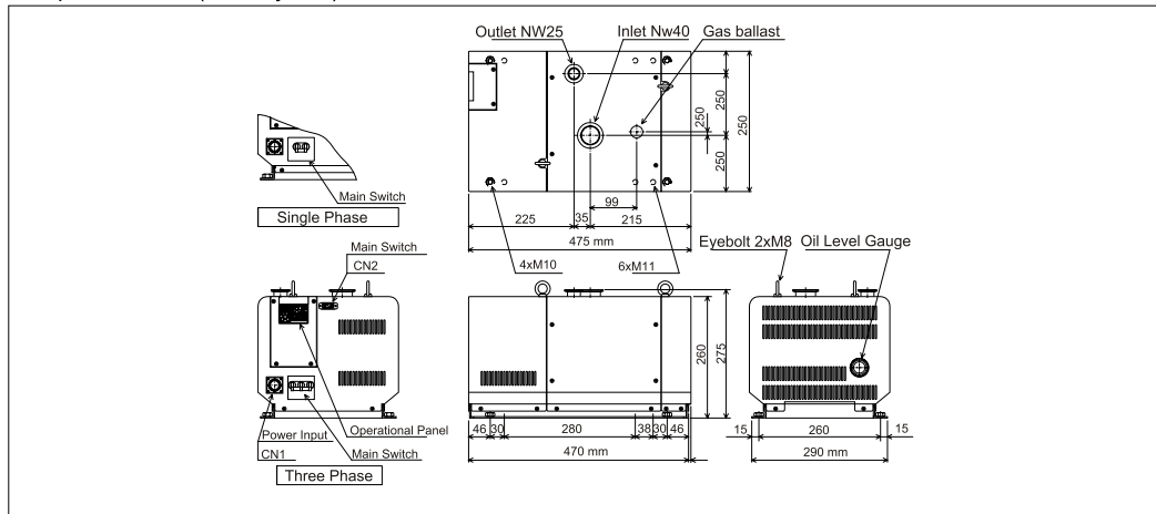
PumpSchematics(NeoDry36C)
