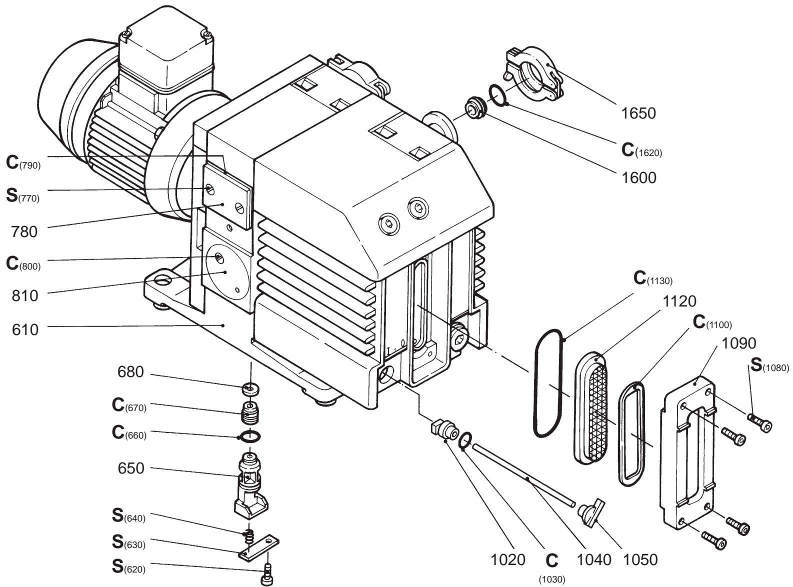
Abb./Fig. 1 TRIVAC D 4/8 B mit Gasballasteinrichtung / with gasballastvalve / avec robinet de lest d'air
